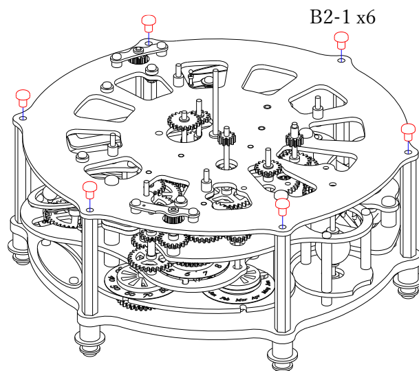
61. 手順 60 のネジを固く締め、同様に 6 ケ所のネジも固く締めます。
