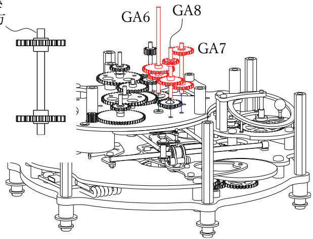
45. 水星駆動歯車 GA6、月を駆動する歯車 GA7 (上図参照)、金星駆動歯車 GA8 を組み付けます。
