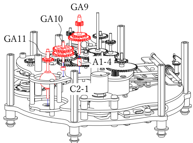
47. 火星駆動歯車 GA9、月相歯車 GA11 および GA10 を組み付けます。(GA11 の月相が下にずり落ちる場合がありますが後の工程で接着するので問題ありません)
